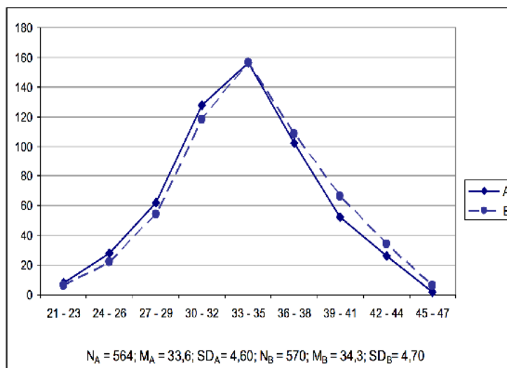
Slika 1. Distribucije rezultata dviju skupina učenika. Rezultati su dobiveni primjenom perceptivnog testa.
